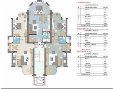
Plan, Etaj 3, Cota: +6.000, Scara 1:100
