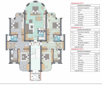
Plan, Etaj 2, Cota: +3.000, Scara 1:100
