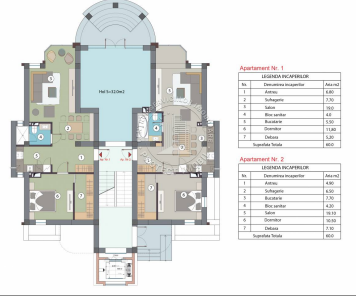
Plan, Demisel, Cota: 3.000, Scara 1:100
