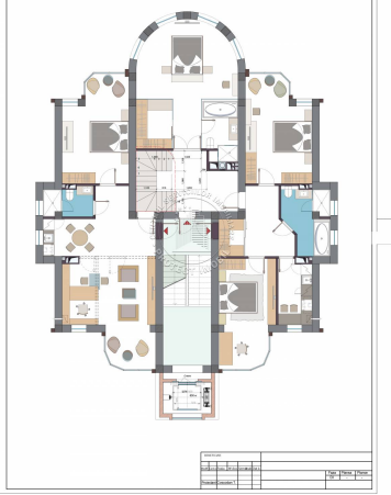
Plan, Etaj 4 Cota +9.000, Scara 1:100
